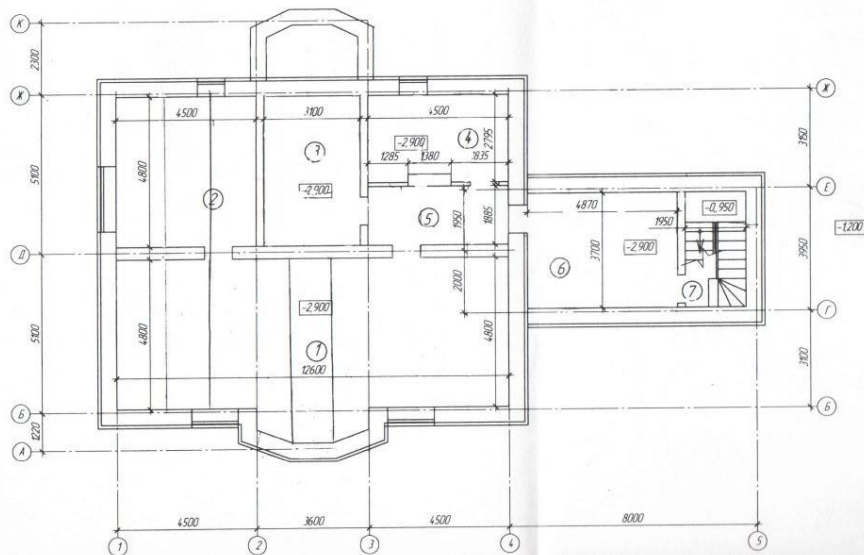
План на отметке -3.000.
