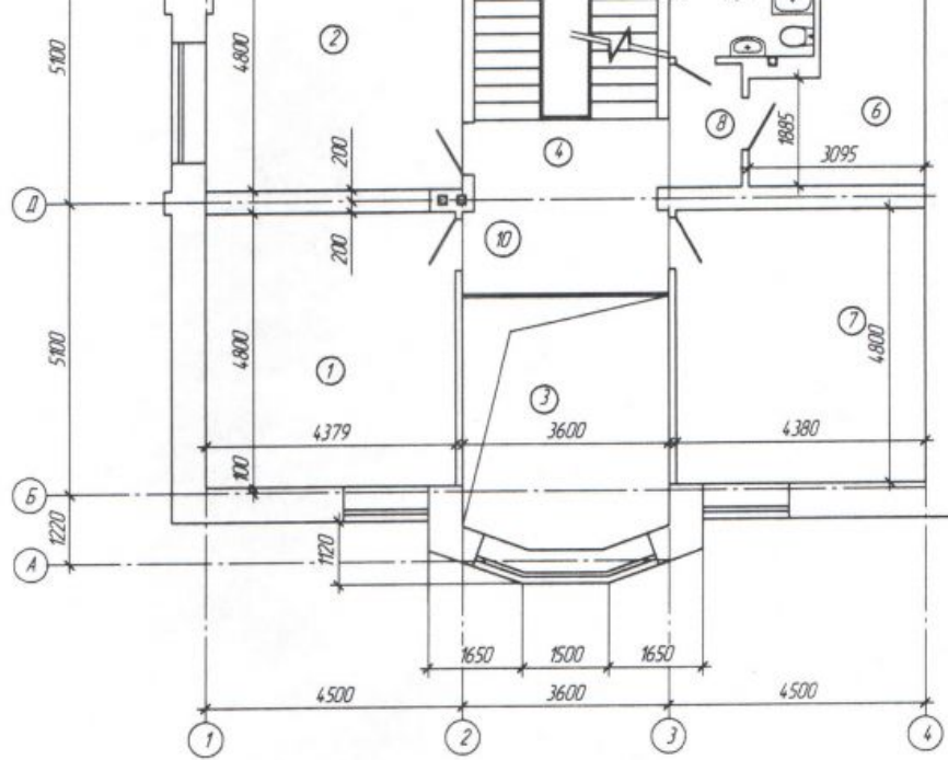
Экспликация помещений на отм. +3.000.
